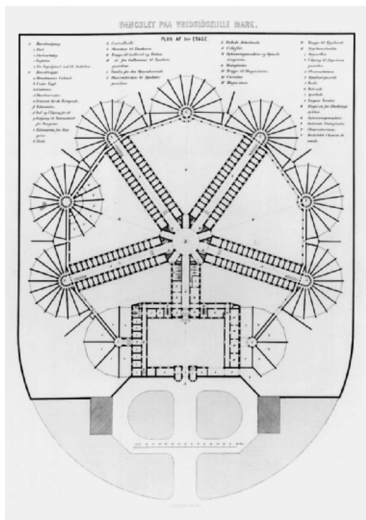
Grundplan af statsfængslerne i Vridsløselille (tv.) og Horsens (th.). Arkitektonisk set var Auburn-fængsler relativt traditionelle bygninger, mens pennsylvanske institutioner var spektakulære panoptiske konstruktioner, der betegnede et nybrud inden for bygningshistorien. Førstnævnte er her illustreret ved grundplanen af Horsens Statsfængsel, der åbnede 1853. Kendetegnende ved Auburn-systemet var de mange små natceller (mærket t) og de store sale, hvor det fælles arbejde udførtes i tavshed (mærket l). Et pennsylvansk fængsel, her illustreret ved Vridsløselille
